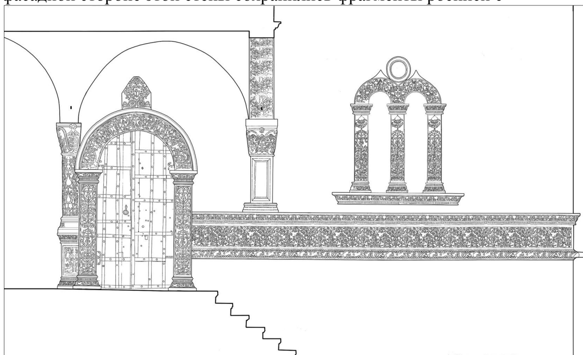
10. Реконструкция северной стены крыльца на 1550-е гг. Чертеж Г.С. Евдокимова и А.М. Дзисько
