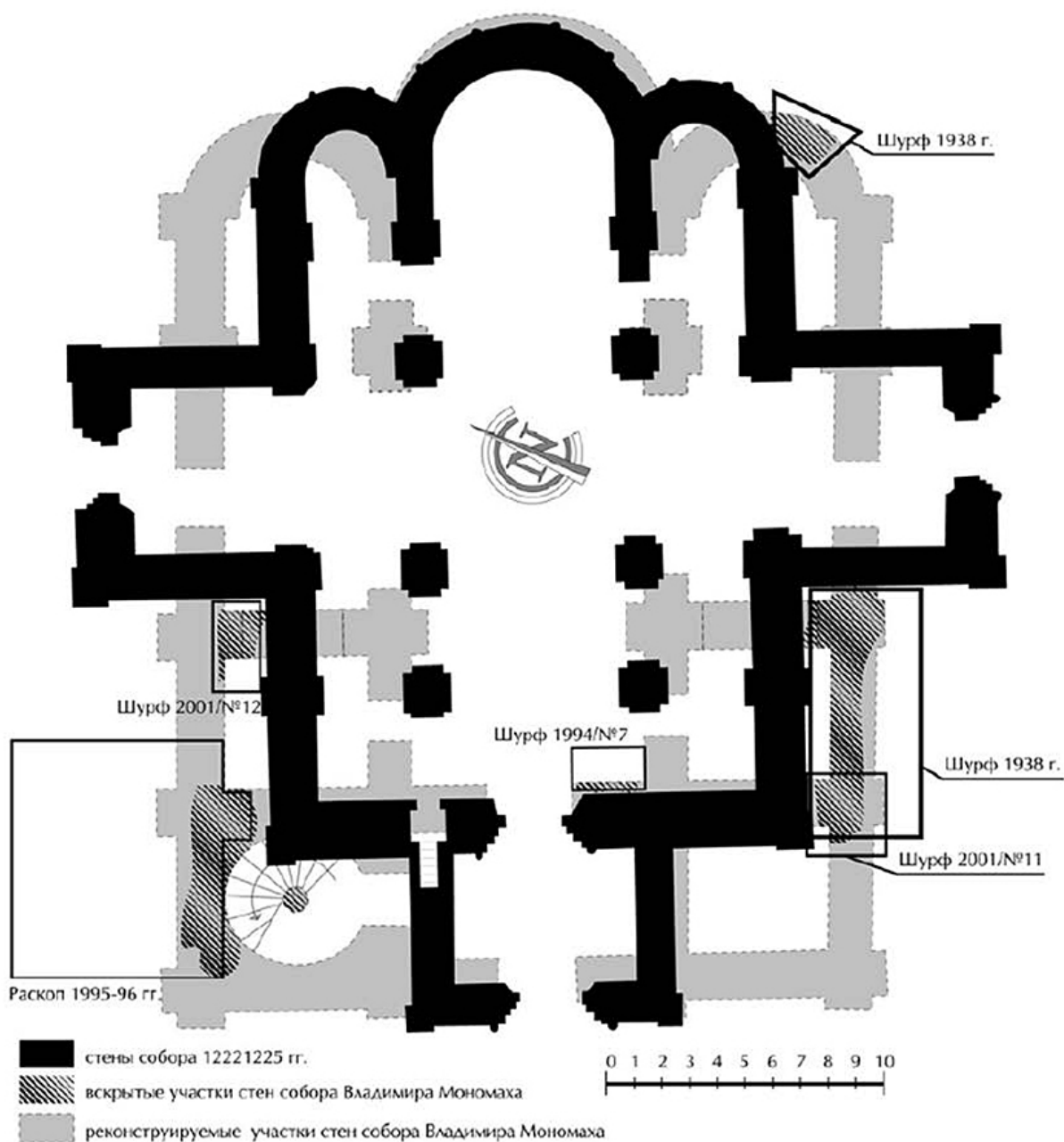
СУЗДАЛЬ. СОБОР РОЖДЕСТВА БОГОРОДИЦЫ. СХЕМА РАСПОЛОЖЕНИЯ ШУРФОВ.
